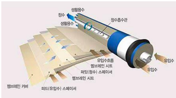
그림 5. 정수기 필터(역삼투압)
